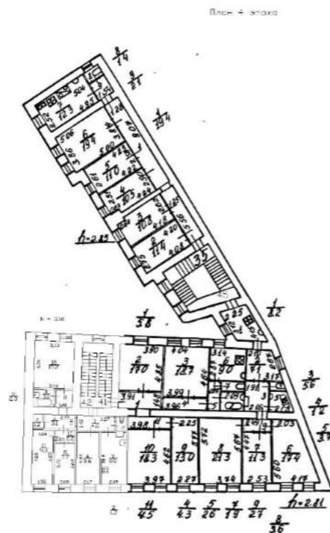
Рис. 5. План 4-го этажа.
